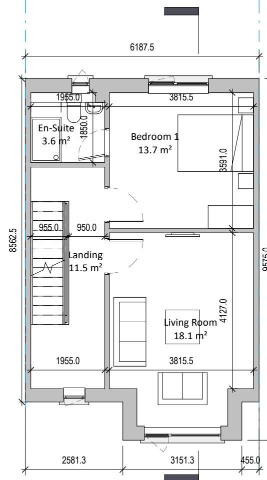
③ H08 Level 01 (MT) 1 : 100
