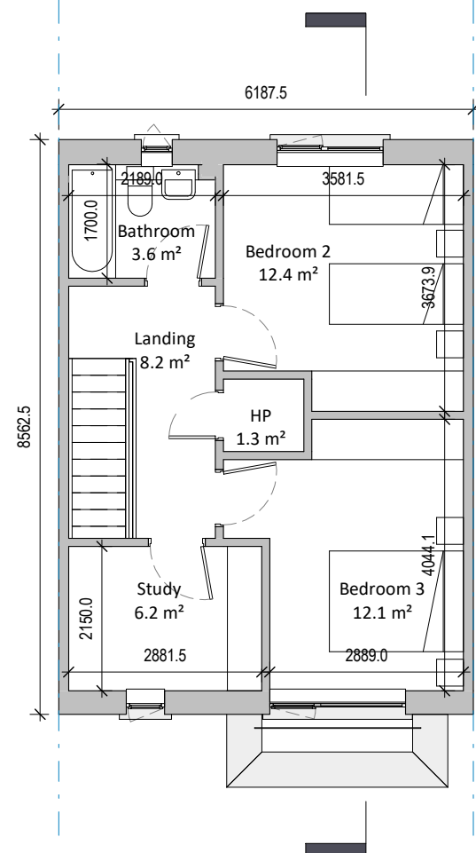
④ H08 Level 02 (MT) 1 : 100
